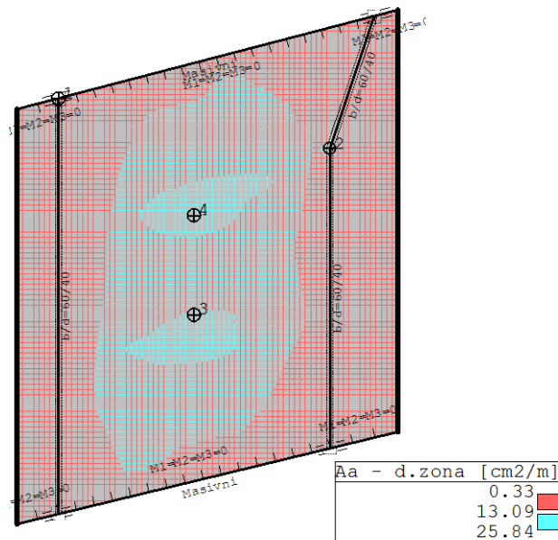
Слика 5 – Дијаграм потребне арматуре у доњој зони плоче новопроектваног моста Figure 5 – Diagram of required reinforcement in lower zone of slab of newly designed bridge
