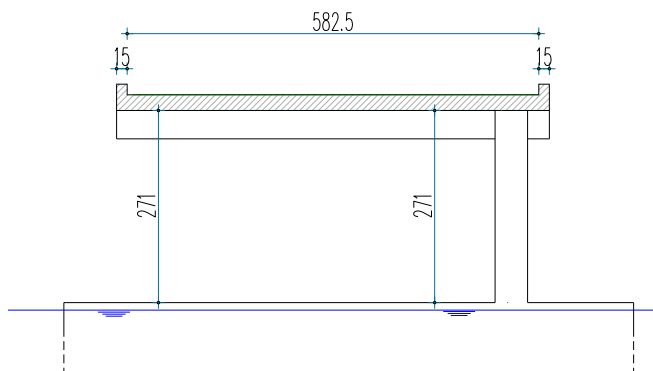
Слика 1 – Попречни пресек постојећег моста Figure 1 – Cross-section of the existing bridge
