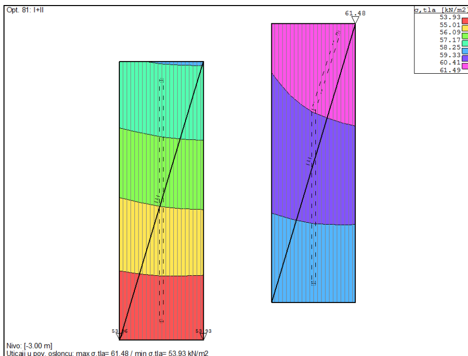
Слика 8 – Максимални напони у тлу [kN/m 2 ] Figure 8 – Maximum stresses in soil [kN/m 2 ]
