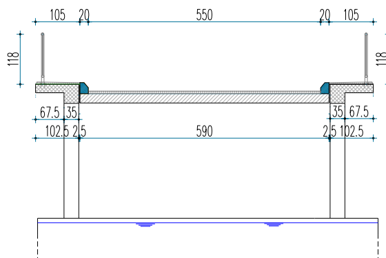
Слика 2 – Попречни пресек новопроектваног моста Figure 2 – Cross-section of the newly designed bridge
