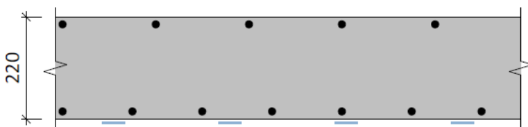
Слика 6 – Распоред трака у попречном пресеку Figure 6 – Arrangement of strips in cross section
