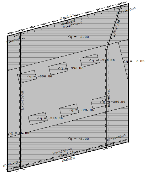
Слика 4 – Шема саобраћајног оптерећења - возило V600 Figure 4 – Traffic Load Scheme - V600 Vehicle
