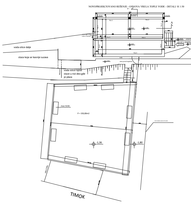
Слика 13. Основа Базена проточне топле воде са плажом
