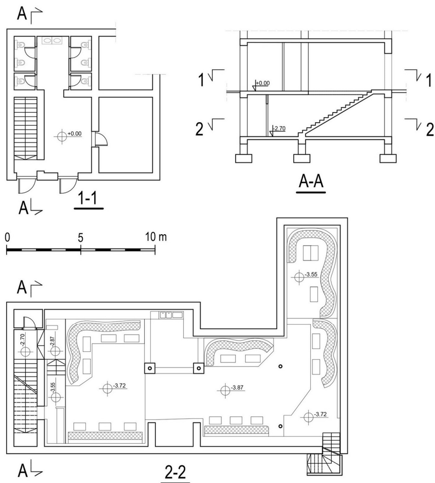
Сл.1 – Основе и пресек ноћног клуба „The Box“
